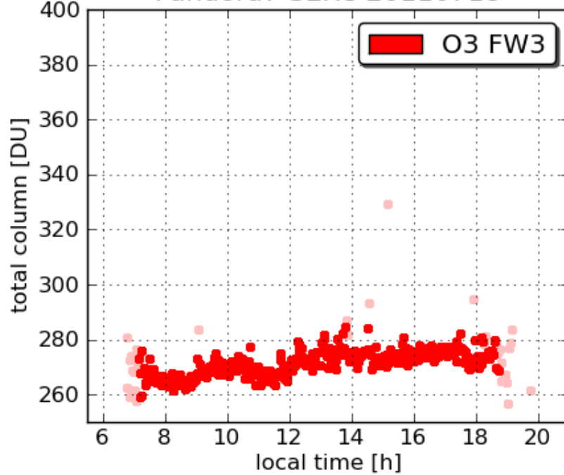
Pandora7 SERC 20110718
