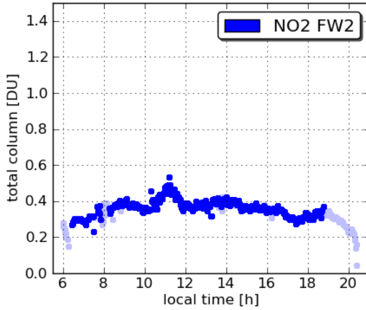
Pandora2 UMBC 20110718
