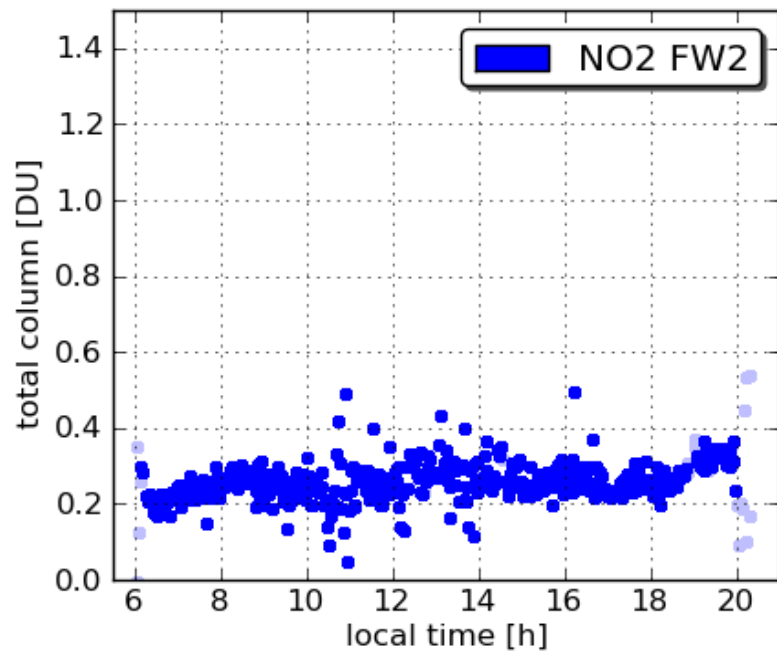
Pandora7 SERC 20110718
