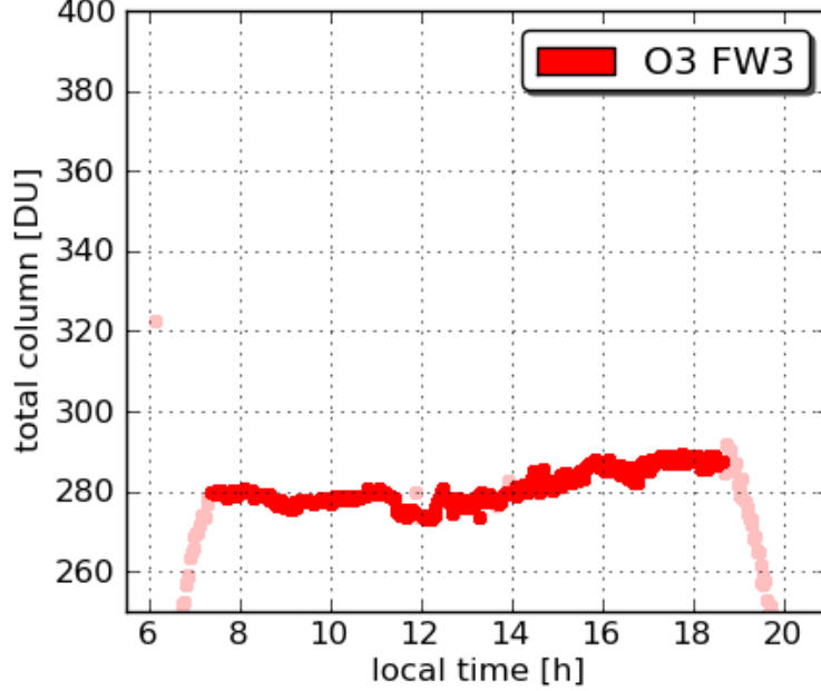
Pandora17 Padonia 20110718
