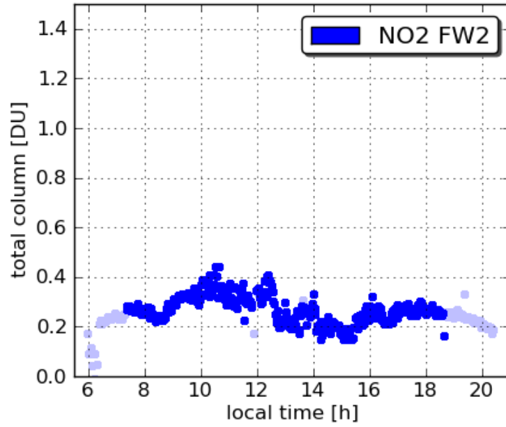
Pandora17 Padonia 20110718
