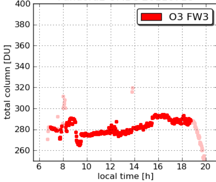
Pandora2 UMBC 20110718
