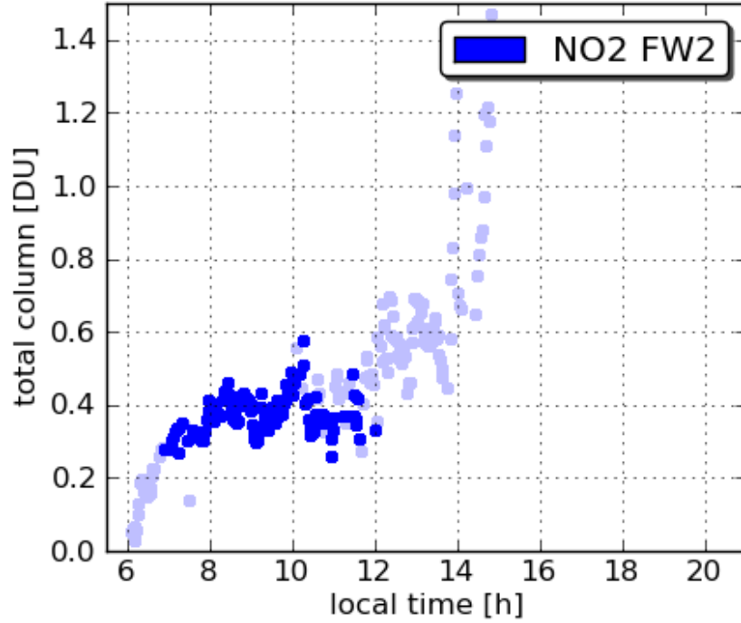
Pandora21 UMCP 20110725
